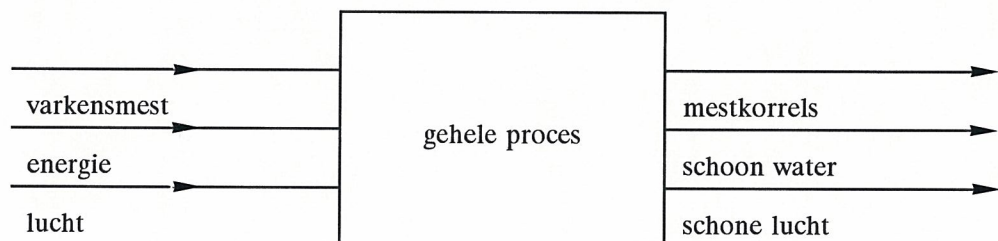
Figuur c Samengevat processchema
